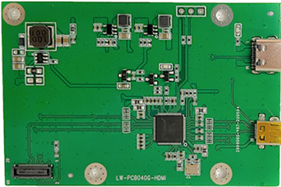
MINI HDMI to MIPI
